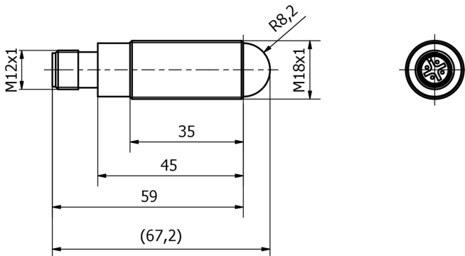
尺寸图 EZ180420
