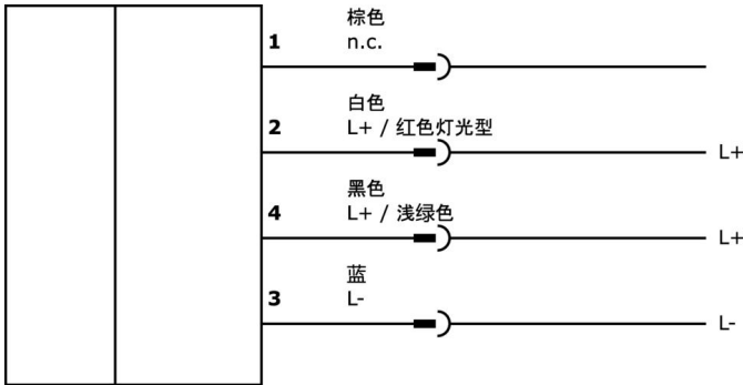
Anschlussbild_EZ180420
